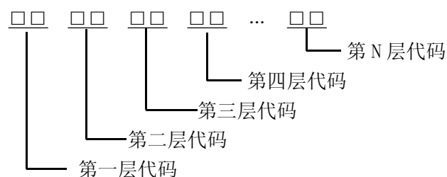
图 1 代码结构图
