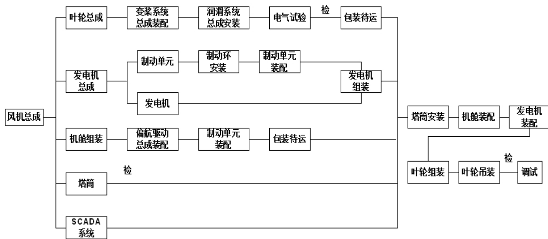
图 1 低风速风力发电机组生产工艺流程图
